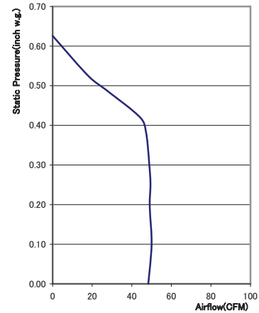
Fan Curve FV-05VK1
