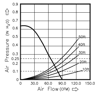
Fan Curve
